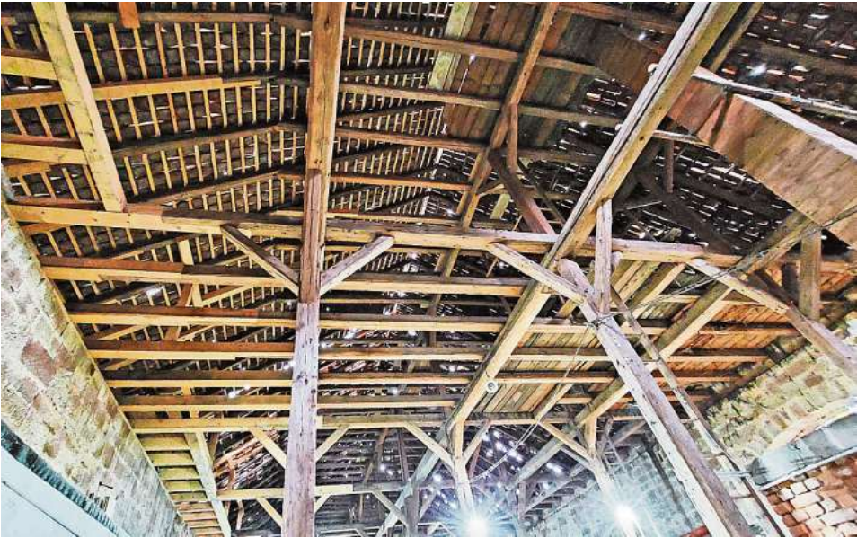
Der Blick zum Scheunendach zeigt, wie viele Balken und Latten hier vor allem auf der linken Seite, zur Marienkirche hin, ausgetauscht werden mussten. Das neue Holz ist heller. Das Dach galt teilweise als einsturzgefährdet.
